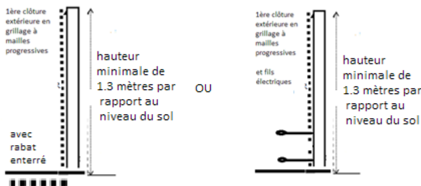
Schéma 1 : Vue de profil des clôtures extérieures décrivant les spécifications techniques minimales permettant d'éviter toute intrusion de suidés sauvages
